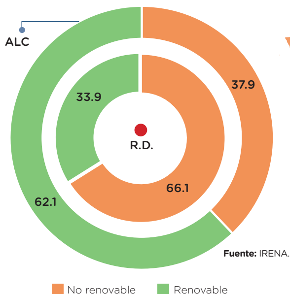
Capacidad instalada de electricidad, 2023 (%)
